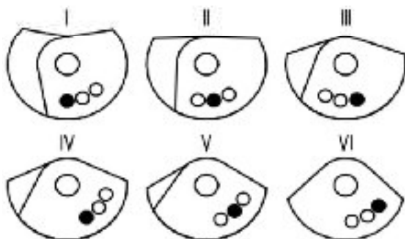
Рис. 3. – Схема регулировки статического момента вибратора (ИБ-98Б)
