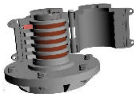
Рис. 5. – Кольцевой токосъёмник
