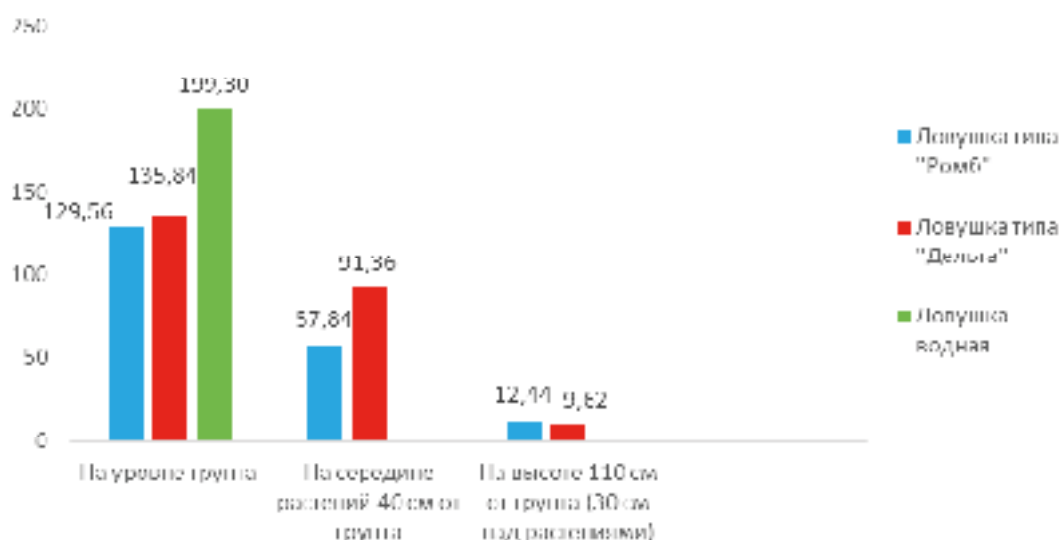
Рис. 5. – Сравнительная диаграмма отлова томатной моли Tuta absoluta различными ловушками на разных уровнях
