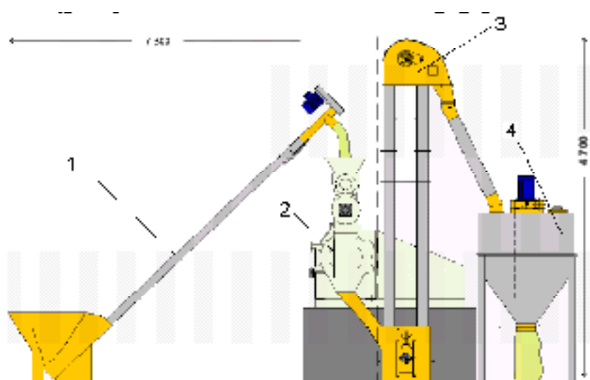
Rys. 8. Linia technologiczna do granulacji pasz z wykorzystaniem przenośnika kufelkowego do załadunku: 1 – przenośnik ślimakowy, 2 – granulator, 3 – przenośnik kufelkowy, 4 – silos na granulaty z wentylacją [materiały informacyjne firmy ELECTRA]
