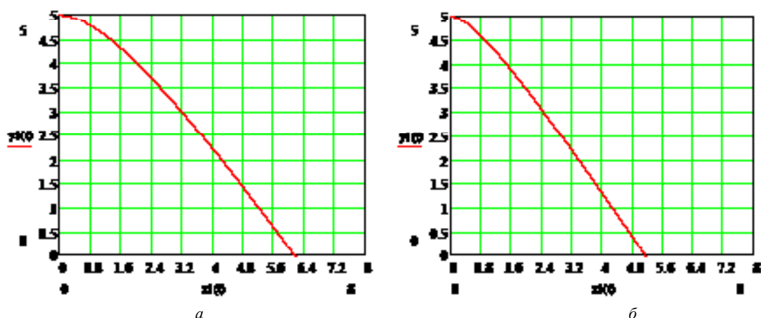
Рис. 2. – Траектория движения частицы биоматериала в зависимости от скорости витания: а – скорость витания 1,5 м/с; б – скорость витания 0,5 м/с
