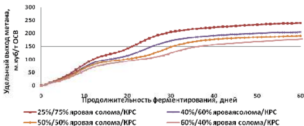
Рис. 2. – Динамика удельного выхода метана с нарастающим итогом, выделившегося при анаэробной ферментации образцов соломы ярового рапса в смеси с навозом КРС в различных соотношениях по ОСВ
