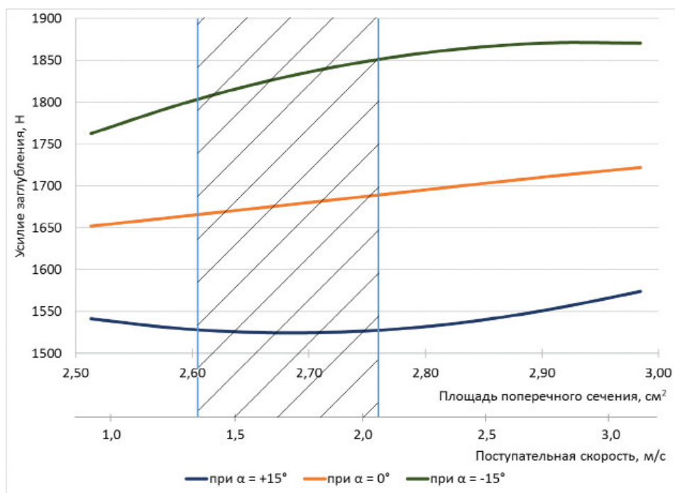
Рис. 3 – График зависимости усилия заглубления пробоотборного зонда от поступательной скорости движения и от площади поперечного сечения зонда
