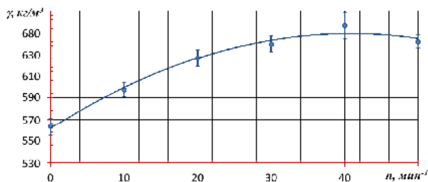
Рис. 8. – Зависимость плотности силосной массы от частоты вращения дебалансов при нормальном удельном давлении 4800 кг/м 2 и статическом моменте дебаланса вибратора 7,7 кг·см (после релаксации)
