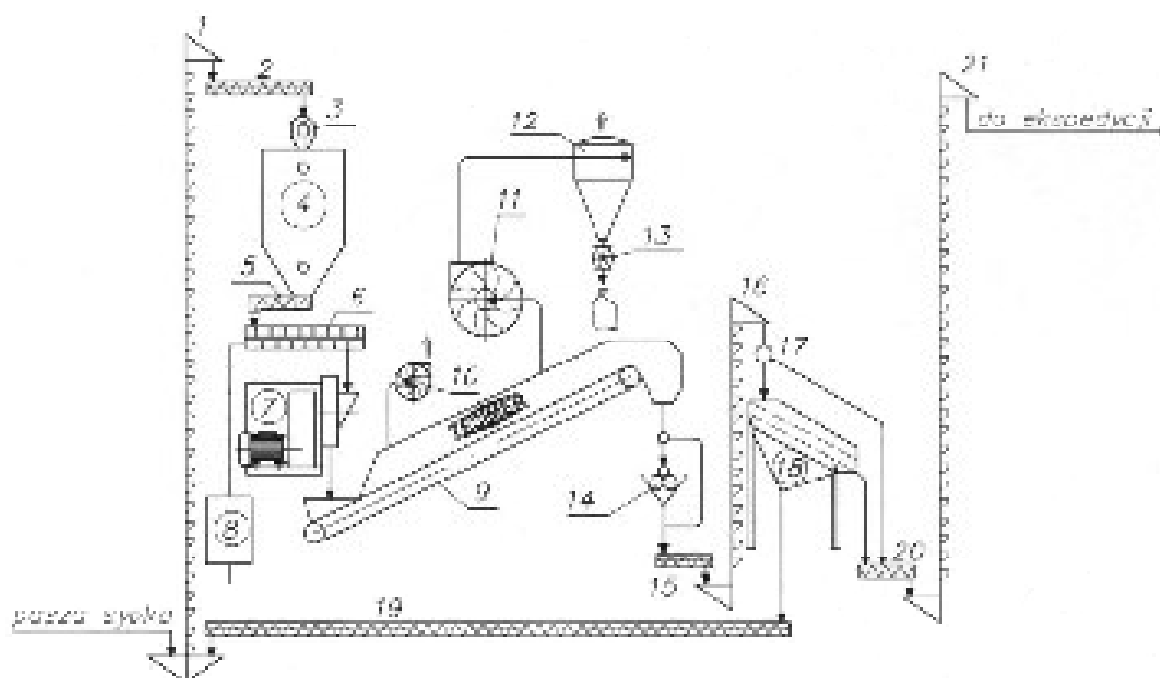
Rys. 10. Linia do granulacji pasz sypkich firmy TESTMER: 1 – podnośnik kubelkowy, 2 – przenośnik ślimakowy, 3 – wychwytywacz magnetyczny, 4 – zbiornik operacyjny nad granulatorem, z czujnikiem minimalnego i maksymalnego napełnienia, 5 – dozownik ślimakowy, 6 – kondycjoner, 7 – prasa granulacyjna, 8 – kocioł parowy lub wytwornica pary, 9 – chłodnica pozioma przenośnikowa, 10 – wentylator aspiracyjny wstępny, 11 – wentylator aspiracyjny główny, 12 – cyklon, 13 – śluza podcyklonowa, 14 – kruszarka granulatu, 15 – przenośnik ślimakowy, 16 – przenośnik kubelkowy, 17 – rozdzielacz dwudrogowy sterowany elektrycznie, 18 – odsiewacz wibracyjny okruszyn, 19, 20 – przenośnik ślimakowy, 21 – podnośnik kubelkowy [katalogi TESTMER S.A. 2017]
