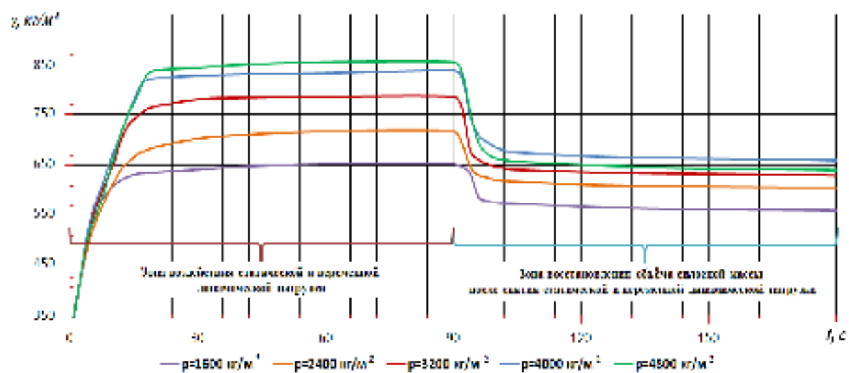
Рис. 6. – Процесс уплотнения силосной массы под воздействием статических и вибродинамических нагрузок ( M_{\text{ст}} = 7,7 \text{ кг} \cdot \text{см} , n = 1800 \text{ мин}^{-1} )
