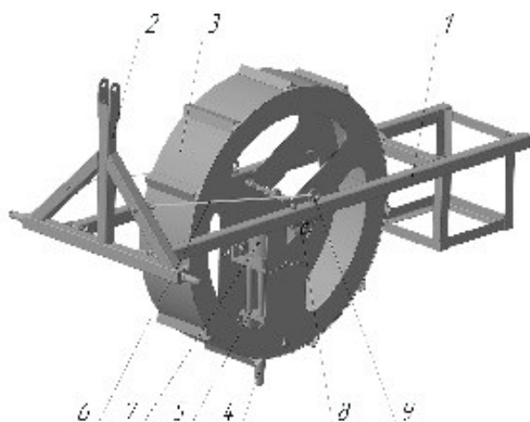
1 – рама; 2 – навесное устройство; 3 – барабан; 4 – пробоотборный зонд; 5 – кронштейн; 6 – тросовый ограничитель; 7 – беспроводной измерительный модуль; 8 – подшипниковый узел; 9 – рым-гайка
