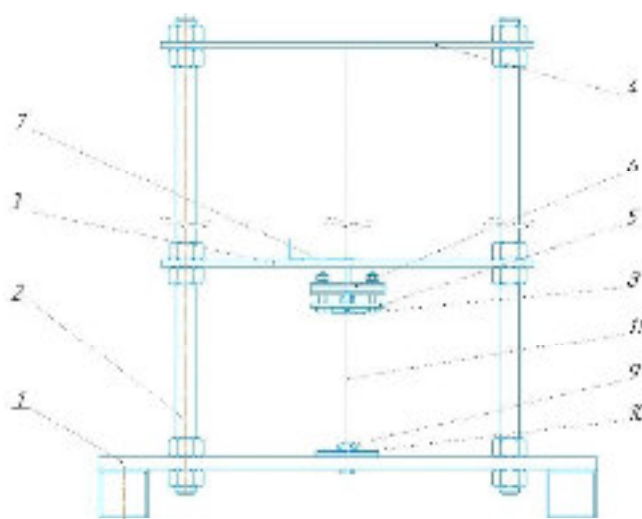
1 – основание; 2 – стойка; 3 – рабочая пластина; 4 – верхняя пластина; 5 – платформа; 6 – груз; 7 – спусковой механизм; 8 – боек; 9 – исследуемое зерно; 10 – предметный столик; 11 – направляющая леска Рис. 1. – Схема (а) и внешний вид (б) стенда для исследования деформации зерна при динамическом воздействии
