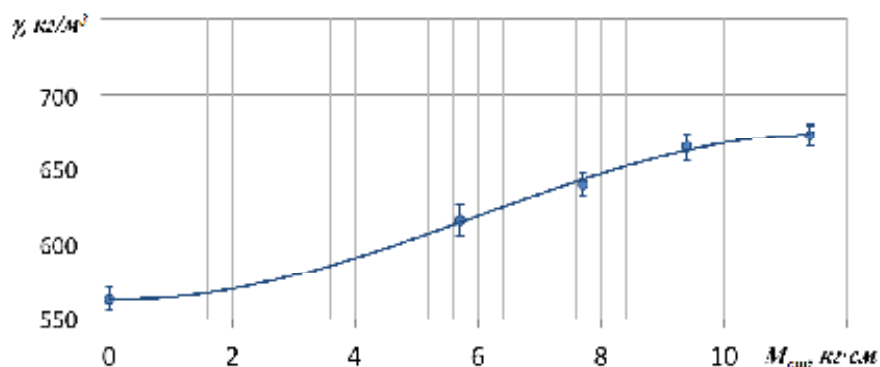
Рис. 9. – Зависимость плотности силосной массы от статического момента дебаланса вибратора при нормальном удельном давлении 4800 кг/м 2 и частоте колебания вибратора 1800 мин -1 (после релаксации)
